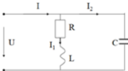
5. ábra. RLC-áramkör, ahol az áram Kirchoff-törvénye értelmében változik.
