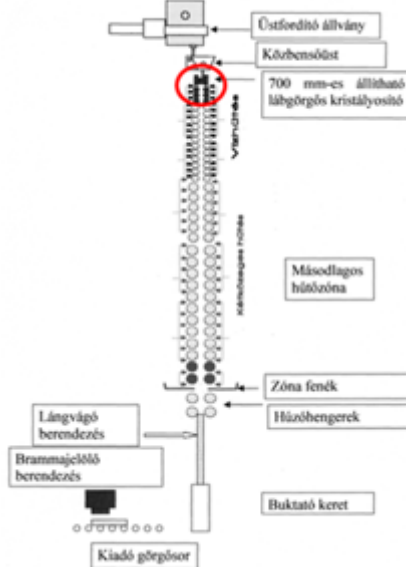
1. ábra. Öntőgép keresztmetszete.
