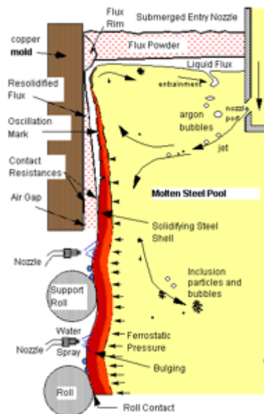
2. ábra. Kristályosítói folyamatok. [1]
